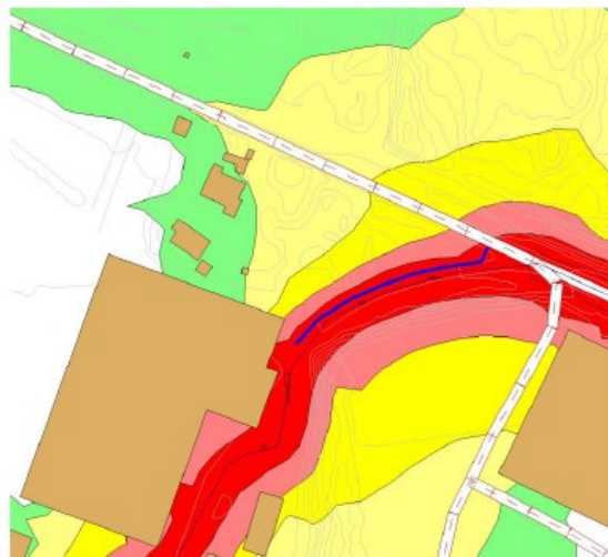
Figur 40 Forslag til støyskjerm langs veien til lagerbygget
