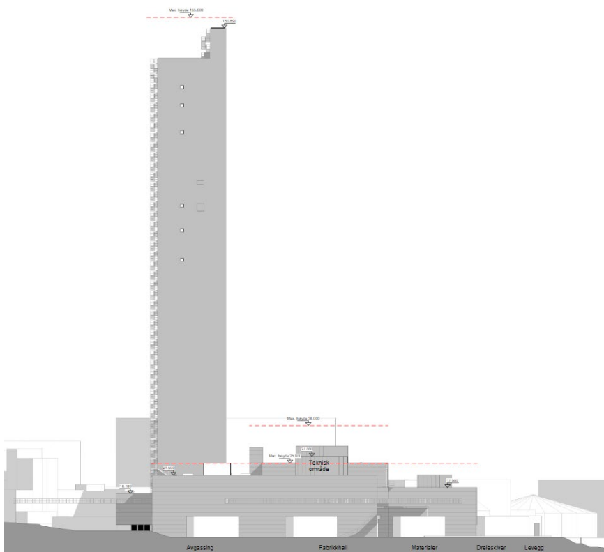
Figur 31 Fasade vest ny bebyggelse i felt B12
