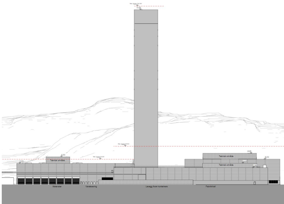
Figur 30 Fasade sør ny bebyggelse i felt B12
