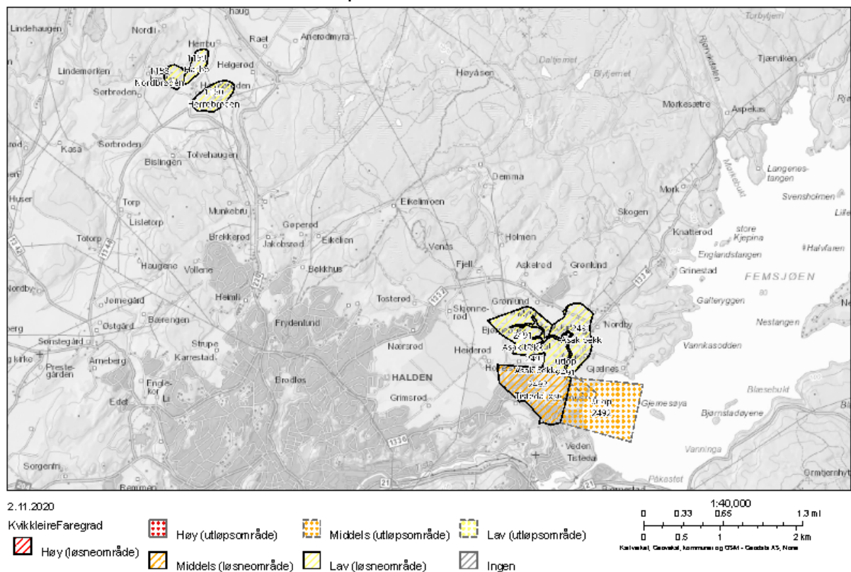
Figur 7 For H210_1 legges farekart i NVE temakart kvikkleire til grunn.
