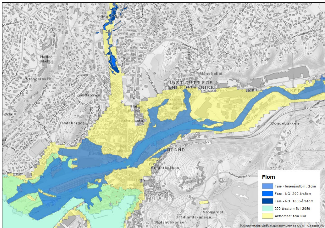
Figur 2 Figuren viser forskjell mellom aktsomhetkart og farekart. Blå farge viser kartlagt fare for flom. Gult felt viser aktsomhetsområde flom. Man kan se at utstrekningen ofte blir mindre når det utarbeides mer detaljerte farekart. Der det finnes farekart skal det legges til grunn, ikke aktsomhetskartet.
