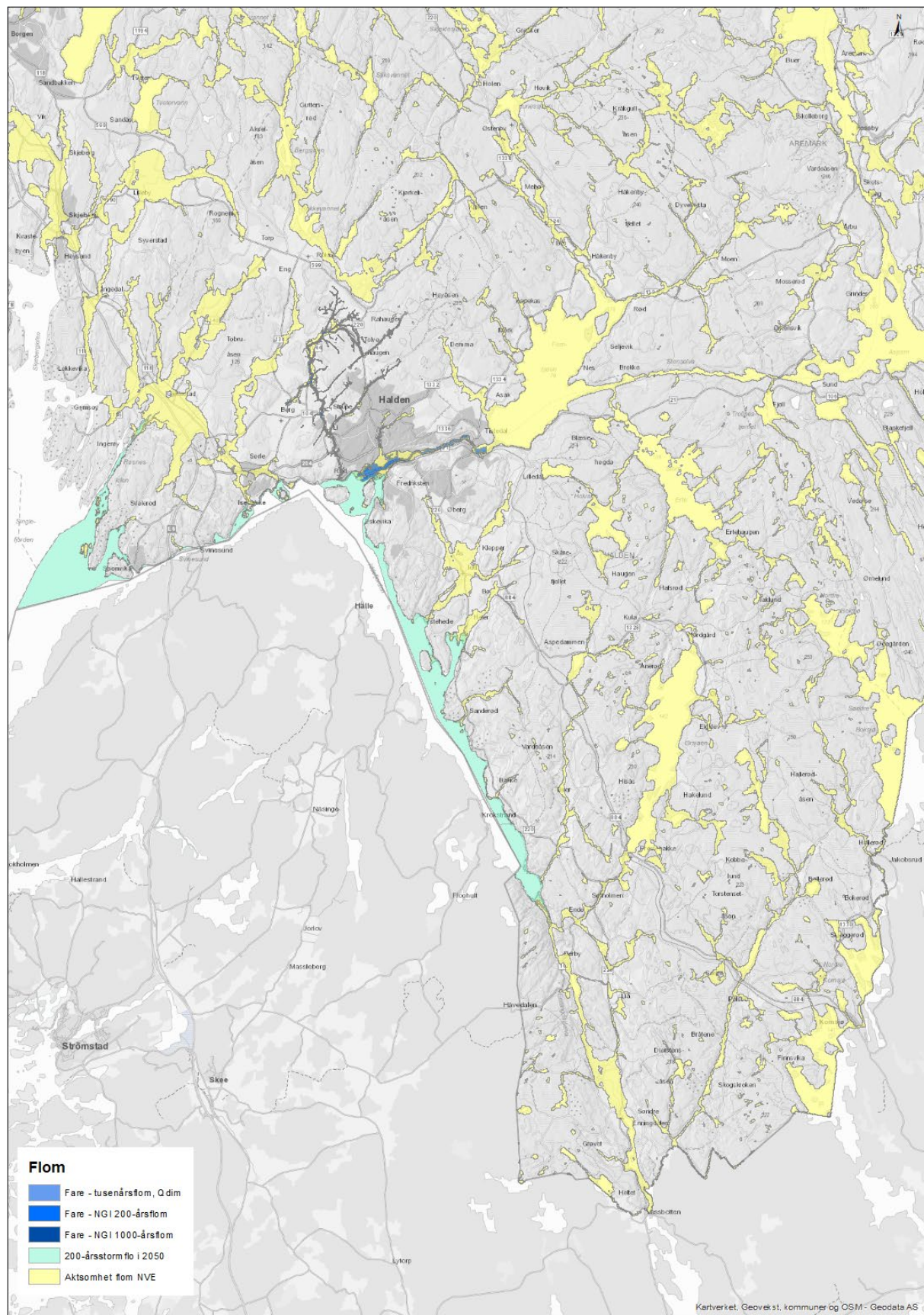
Figur 8 Aktsomhets- og fareområder for flom og stormflo, jf NVE atlas, NGI rapport, kartverkets "sehavnivå" og Haldenvassdragets brugsseierforenings Qdim..
